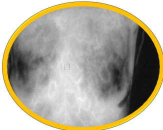
SPY QP
